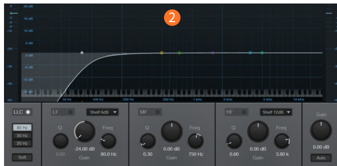
• 图 ② 是高通频率80Hz。Q值0.7曲线。
